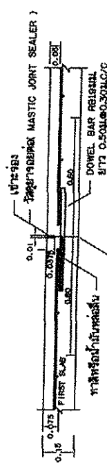
แบบขยายข้อต่อหดตัว
